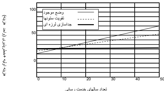
شکل ۵-۱۳- هزینه‌ی اجرا و خطرپذیری زلزله برای یک ساختمان
