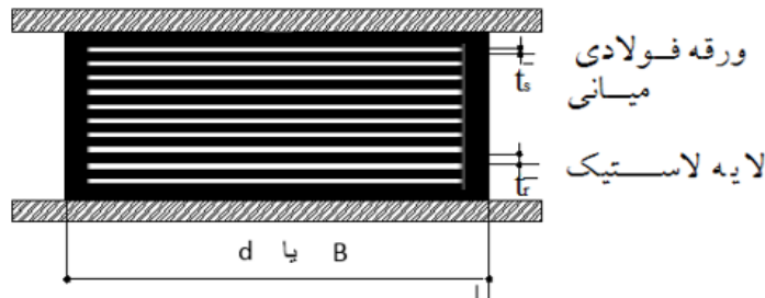
شکل ۳-۵- مقطع جداساز لاستیکی با ورق‌های فولادی
